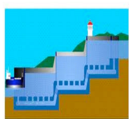
Figura 1: Sistema de esclusas del canal de Panamá.
